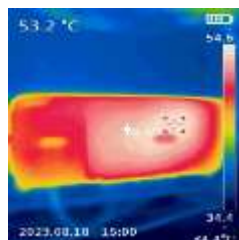
Inverter NO.2 อุณหภูมิ 54.6 °C
