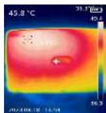
Inverter NO.1 อุณหภูมิ 49.4 °C
