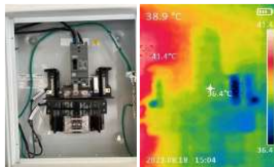
ตู้LP อุณหภูมิ 41.4 °C
